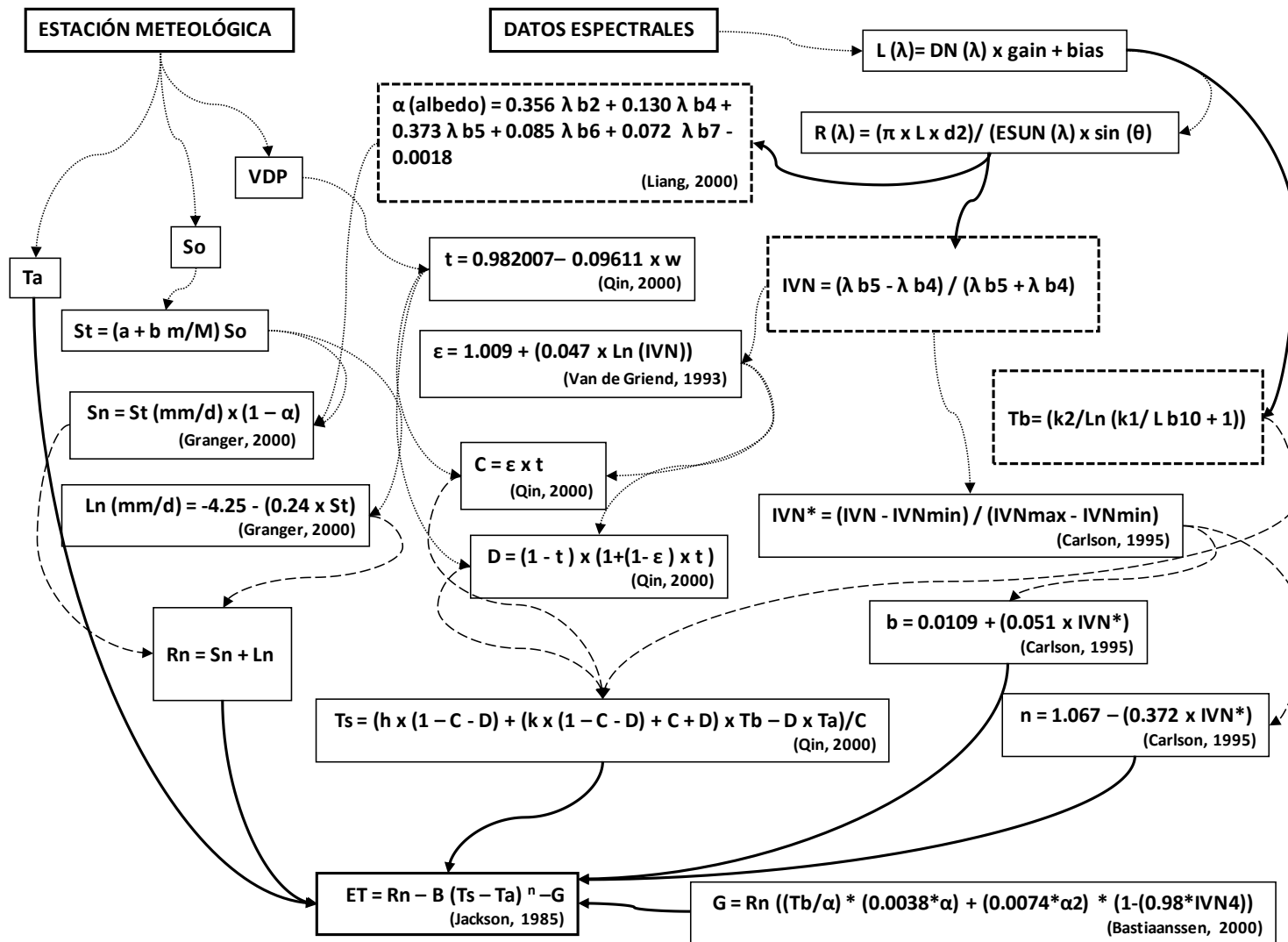
Figura 4.1: Proceso realizado para estimar la evapotranspiración a partir de imágenes Landsat 8 y datos meteorológicos en las 133 micro-cuencas en estudio. Ta: temperatura del aire; So: Radiación solar; VDP: Presión de vapor de agua; St: Radiación de onda corta total entrante; Sn: Radiación neta de onda corta; Ln: Radiación neta de onda larga; Rn: Radiación neta; \alpha : albedo; t: transmitancia; \epsilon : emisividad; C y D: Coeficientes derivados de la emisividad y transmitancia; Ts: Temperatura superficial; L( \lambda ): Radiancia; R( \lambda ): Reflectancia; IVN: Índice de Vegetación Normalizado, Tb: Temperatura superficial por Banda 10 de Landsat 8; IVN*: IVN escalonado; b y n: parámetros derivados del IVN característicos de la vegetación; G: Flujo de energía del suelo y ET: evapotranspiración.
